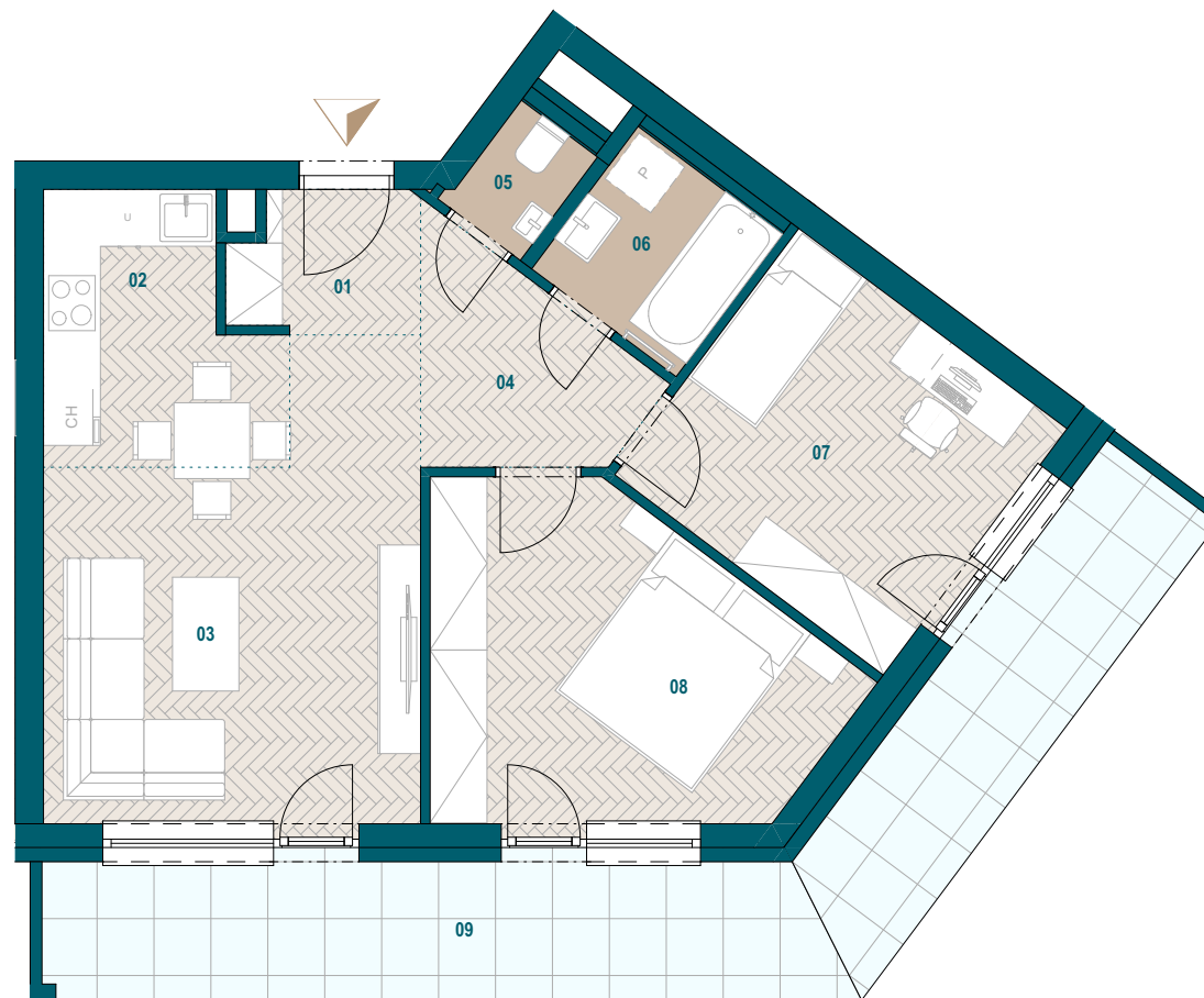
6. nadzemné podlažie
